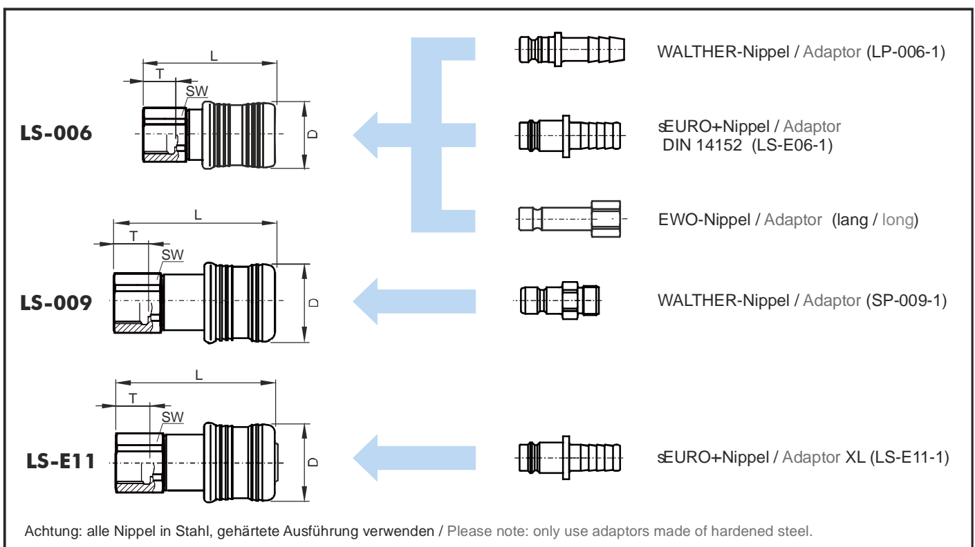
Type LS-006 mit Nippel LP-006 Type LS-006 to Adaptor LP-006
