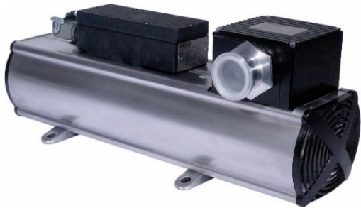
Bild 1 Heliumdichtes Seitenkanalgebläse für Anlagen additiven Fertigung
