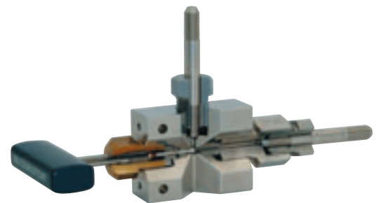
Schnittmodell 2-Wege-Nadelventil
