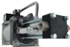
Druckluftnachverdichter Typ GPLV5-Serie
