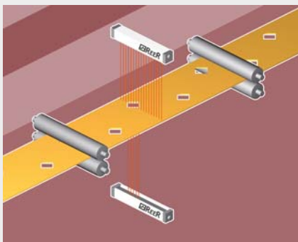
Qualitätskontrolle: Erkennung des Vorhandenseins, der Größe und der Position von Löchern
