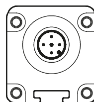
Sender M12 5-polig
