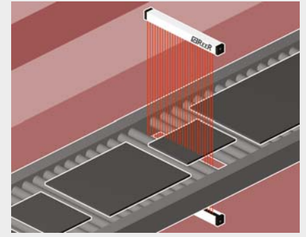
Messen der Breite und Position von Platten auf Transportsystemen
