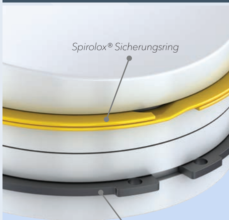
Gewöhnlicher Schnapping (Cirlclip)
