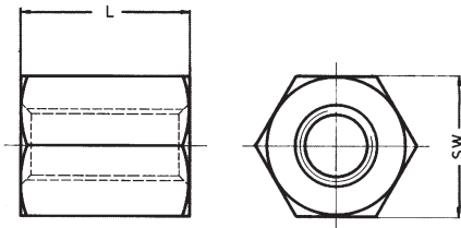
Sechskant-Trapezgewinde-Muttern
