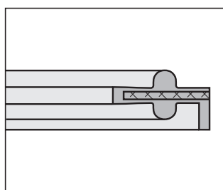
4FC Ausführung E PTFE ummantelte EPDM-Dichtung mit Bund, Abmessungen auf Anfrage Version E PTFE encapsulated EPDM gasket with flange, sizes on request
