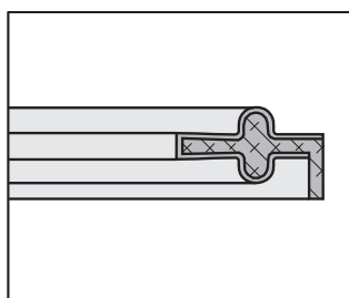
4FC Ausführung D PTFE ummantelte EPDM-Dichtung mit Bund, Abmessungen auf Anfrage Version D PTFE encapsulated EPDM gasket with flange, sizes on request
