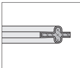
4FC Ausführung C PTFE ummantelte EPDM-Dichtung ohne Bund, Abmessungen auf Anfrage Version C PTFE encapsulated EPDM gasket without flange, sizes on request
