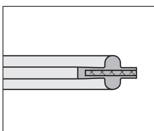
4FC Ausführung F PTFE ummantelte EPDM-Dichtung ohne Bund, Abmessungen auf Anfrage Version F PTFE encapsulated EPDM gasket with flange, sizes on request
