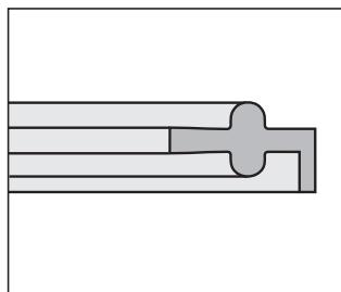
4FC Ausführung A Dichtung mit Bund Version A Gasket with flange
