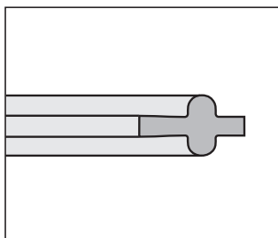
4FC Ausführung B Dichtung ohne Bund Version B Gasket without flange
