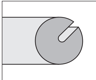
ROD PTFE O-Ring, Schlitz außen um 45° versetzt PTFE O-Ring, 45° outside slot
