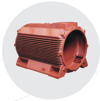
Stator frame 586 kg, EN-GJL-200
