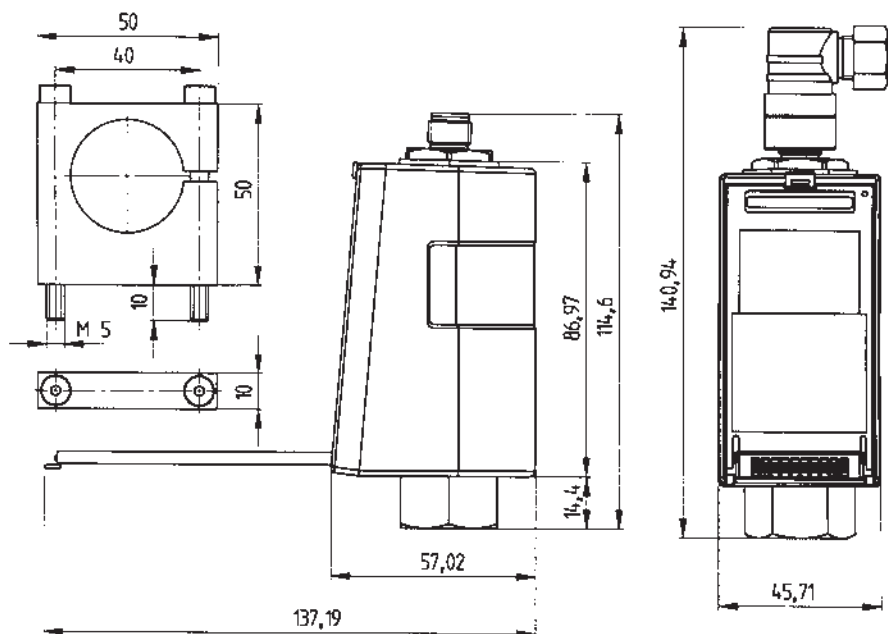
Staffa di fissaggio / Mounting bracket
