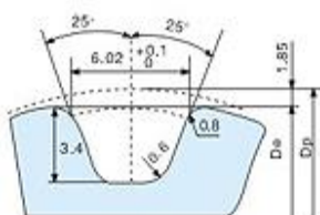
T10型齿形图: Tooth form diagram
