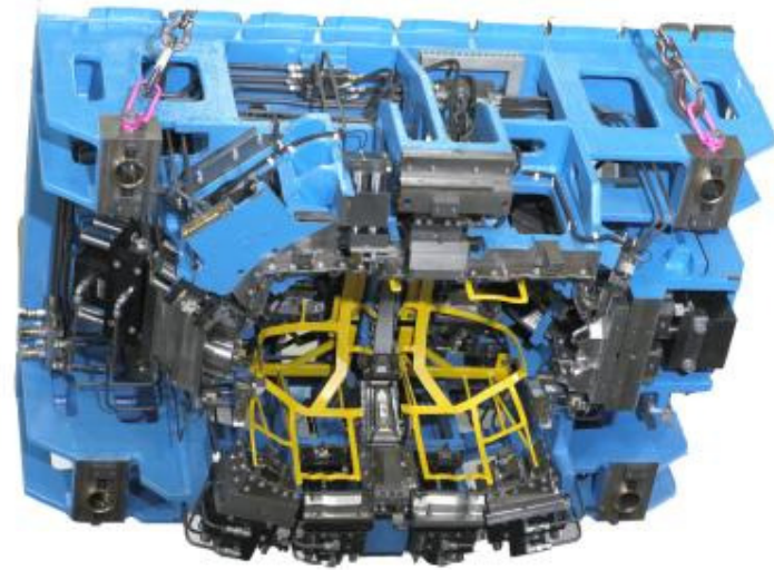
Stanzwerkzeug für textile Radlaufschaale
