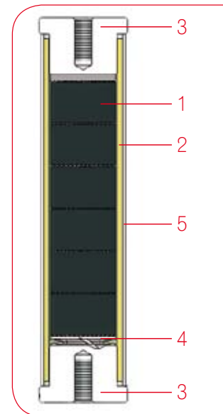
ASW 18 type surge arrester Überspannungsableiter Typ ASW 18
