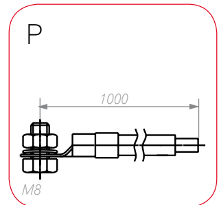
Cu insulated flexible conductor isolierte Cu-Schlauchleitung
