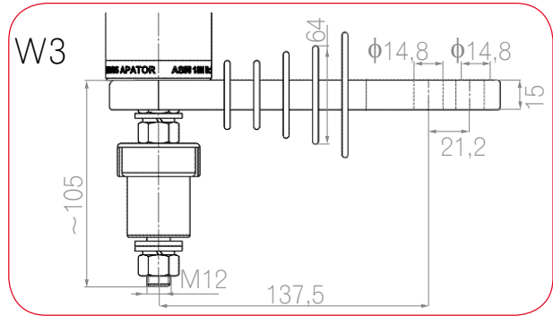
insulating bracket with disconnector Isolationsträger mit einem Trennschalter
