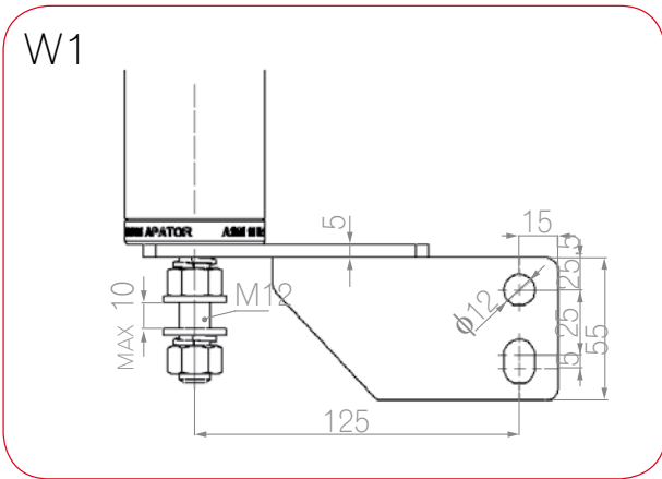
angle metal bracket Einbauwinkel
