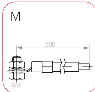
Cu insulated flexible conductor isolierte Cu-Schlauchleitung
