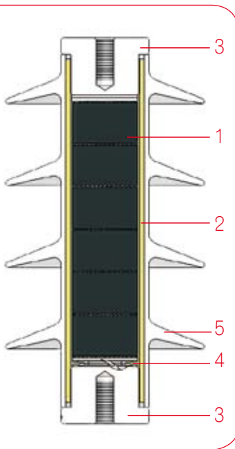
ASM 18N type surge arrester Überspannungsableiter Typ ASM 18N
