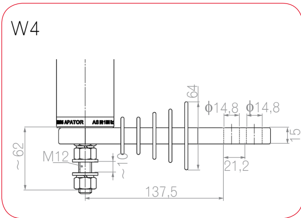
insulating bracket Isolationsträger
