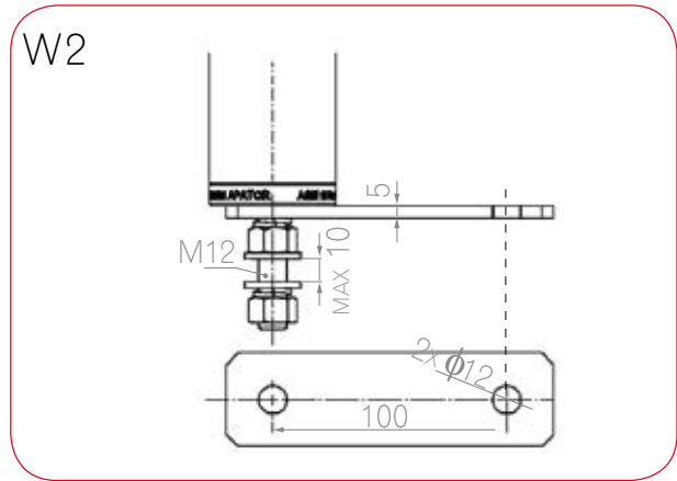
straight metal bracket einfacher Einbauträger
