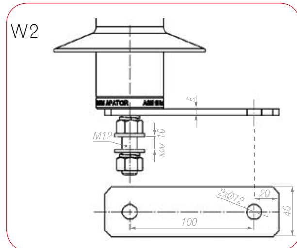
straight metal bracket einfacher Einbauträger
