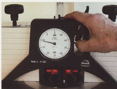
Messen der unteren Schneide
