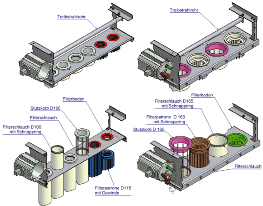
Funktionsprinzip
