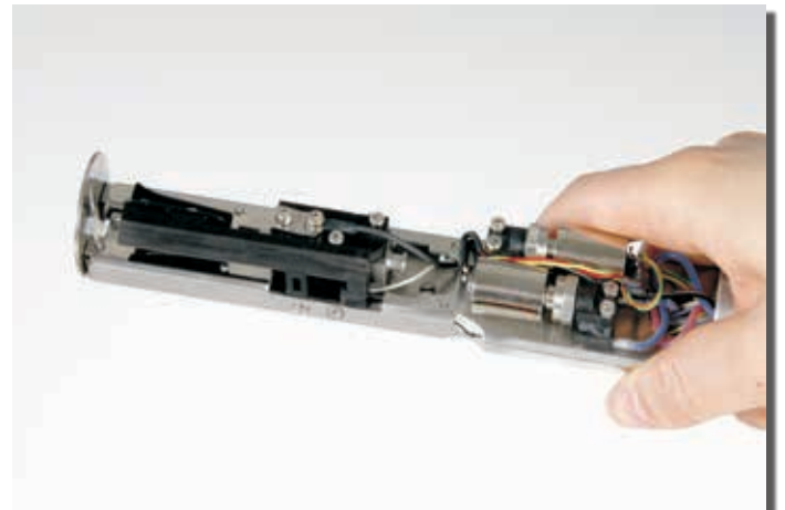
Schreibkopf mit selbstschließenden Ventilen Printhead with locking valves
