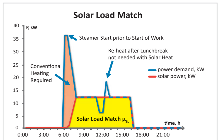
Solarthermische Überdeckung eines Prozeßdampf-Systems Solar Load Match of a Hybrid Process Steam System
