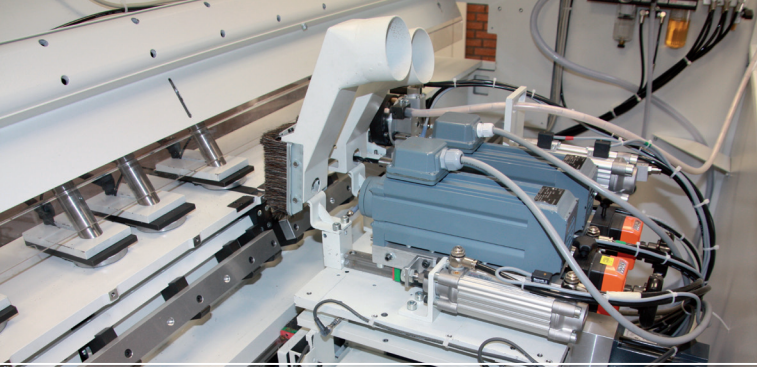
Bohr + Fräsupport mit 2 Fräsaggregaten
