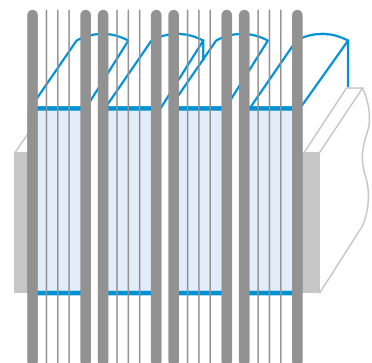
Kanalführung mit je zwei Zerspanersägen
