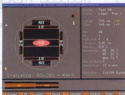
Cutting pattern optimisation
