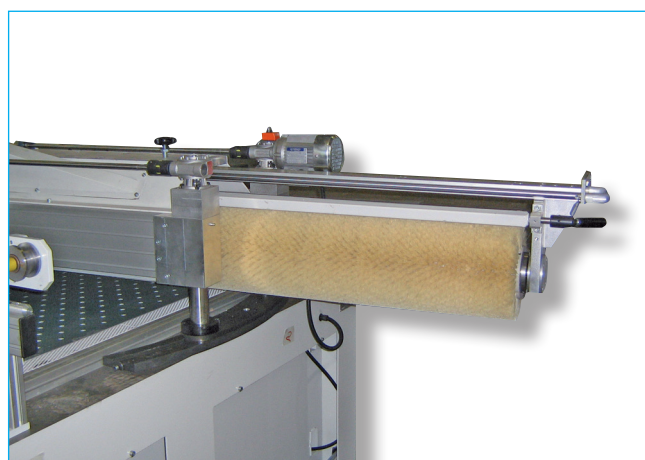
Sistema estraibile della spazzola - Extractable brush system
