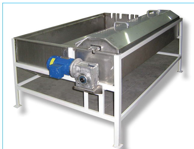
Sistema di pulizia della spazzola - Brush washing device
