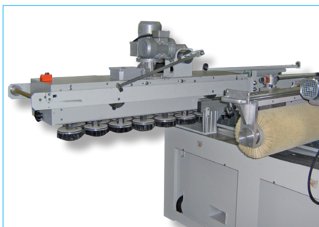
Sistema estraibile dei piattorelli - Wiping disks for transversal veneer
