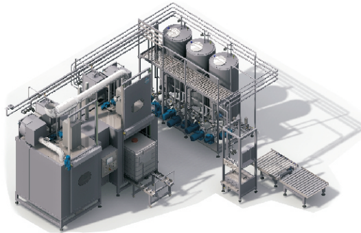
Reinigungs- und Trocknungskabine mit Medientanks Gebinde- Innen- und Außenreinigung mit Umlufttrocknung
