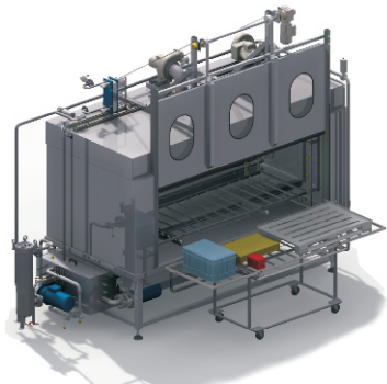
Chargen-Reinigungskabine modulare Baureihe mit dynamischer Düsentechnik für unterschiedliche Reinigungsgüter
