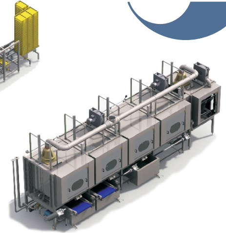
Taktgesteuerte Durchlauf-Reinigungsanlage innovative Prozessmodule mit dynamischen Spritzsysteme bis 120 bar
