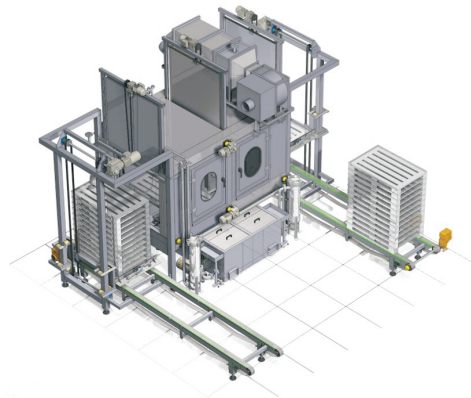
Reinigungskabine mit automatischer Bestückung getrennte Reinigungs- und Trocknungszone mit jeweils kundenspezifischer Linienführung
