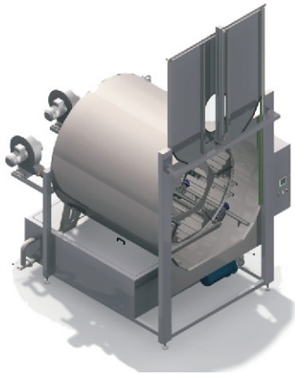
Rhönrad-Reinigungskabine in Hygienic Design mit individuellen Reinigungs- und Trocknungsprozesse
