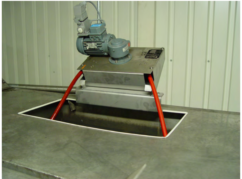
Ölskimmer Modell W40 an Entfettungsbad
