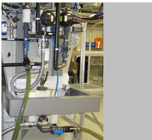
Standard AF Ablaufverteiler Typ 2 mit Armaturen für Tuchspülung im Kreislauf, sowie Automatikarmaturen für Klar- und Trüblauf.
